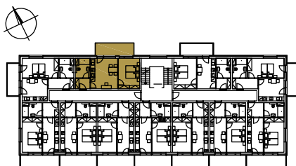
PŮDORYS PATRA
